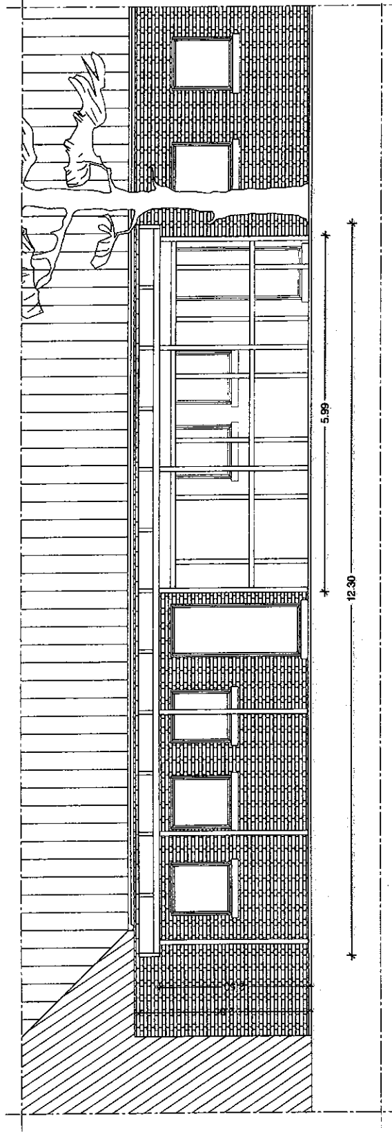
Ansicht Wintergarten / Terrassendach M. 1:50
