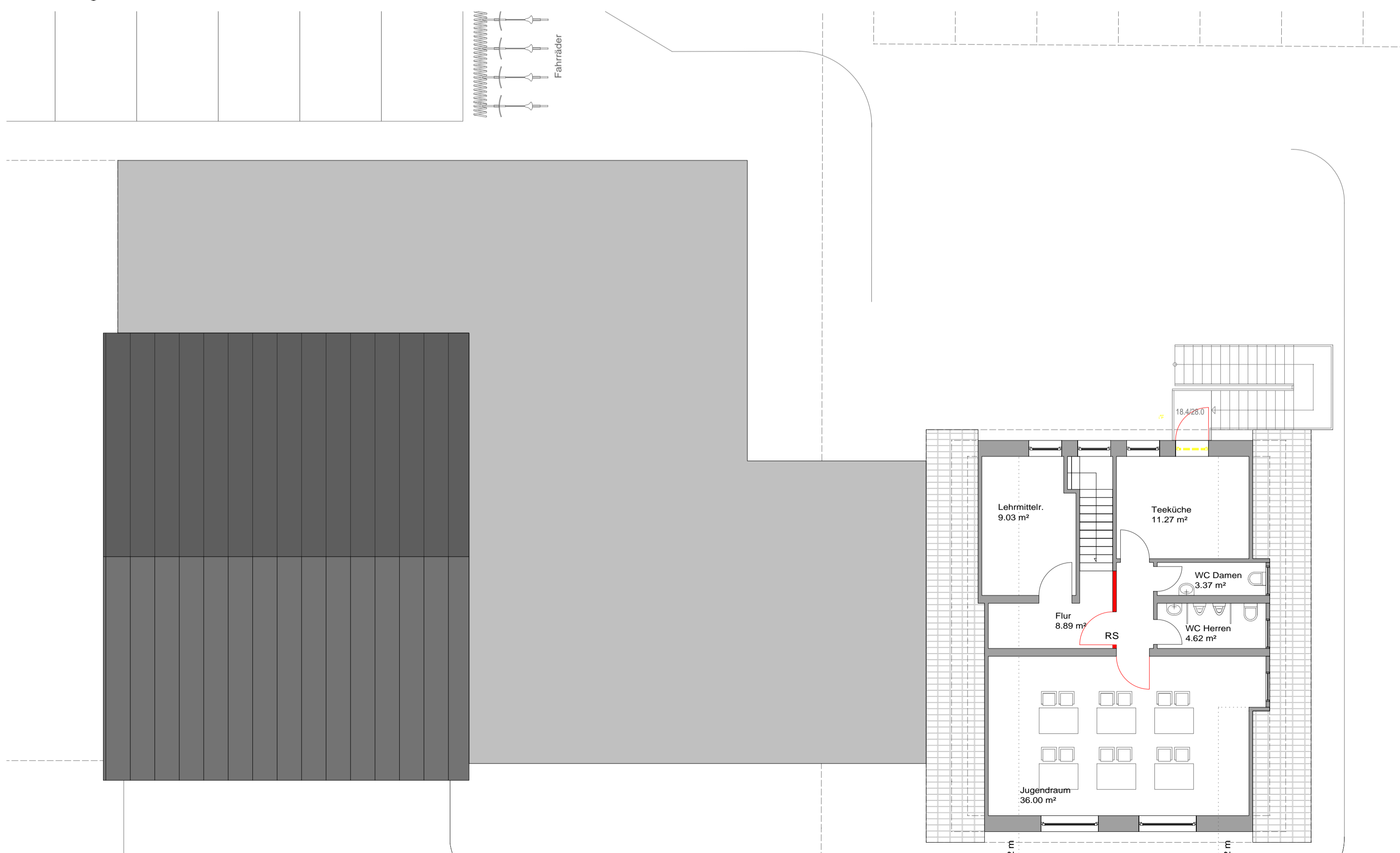
Dachgeschoss m. 1:100
