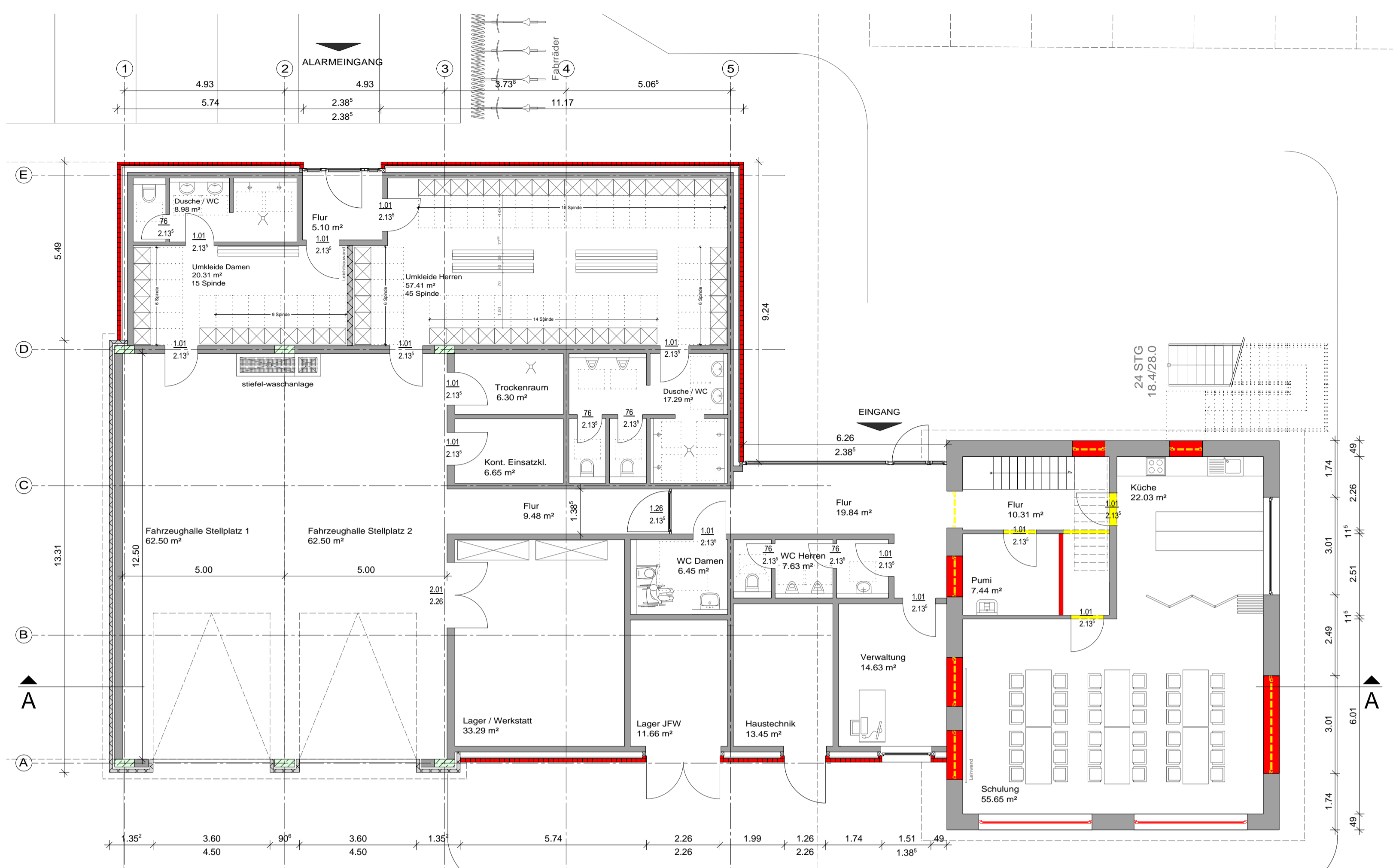
Erdgeschoss m. 1:100
