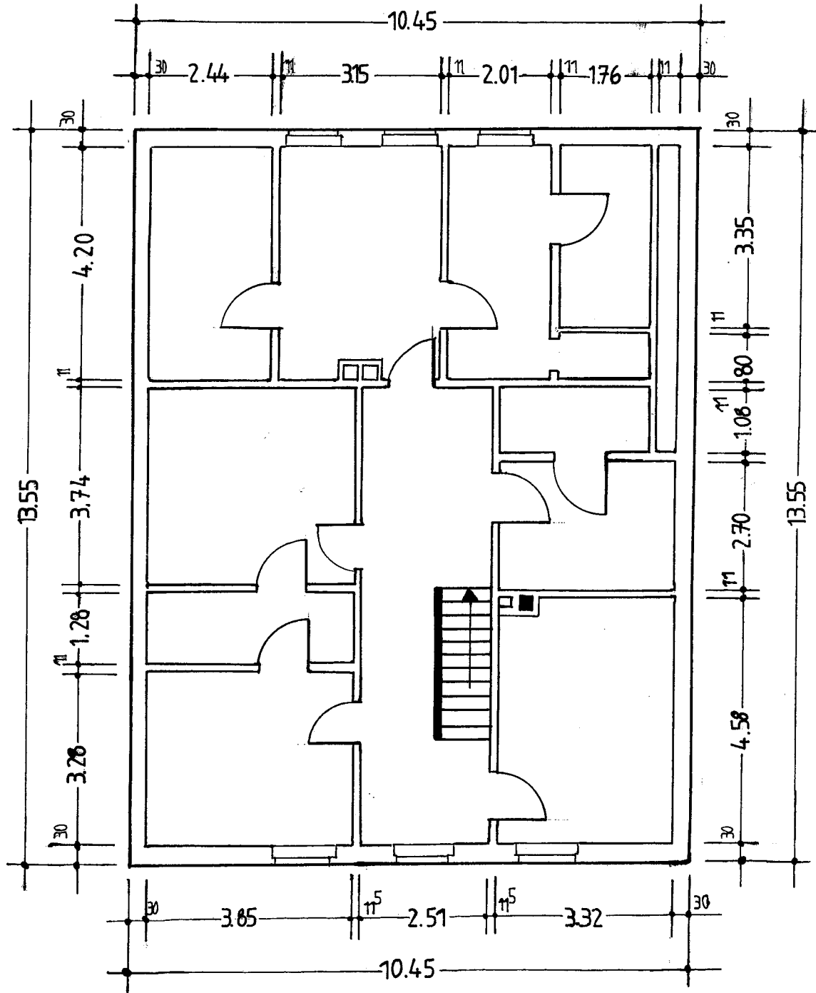
Wohnhaus Marxer Hauptstraße 49 - Grundriß OG - M. 1:100 - 05.02.2010
